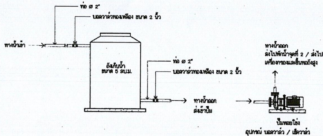
แบบตัวอย่างจุดพักน้ำ No Scale
