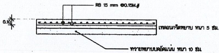
ขยายพื้นวางถังเก็บน้ำ ขนาด 5 ลบ.ม. Scale 1 : 25
