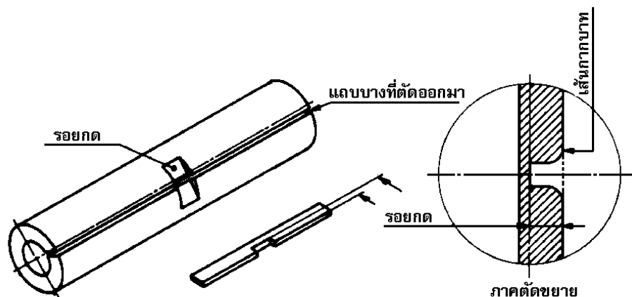
รูปที่ 5 การวัดรอยกด (ข้อ 10.4.5.4)
