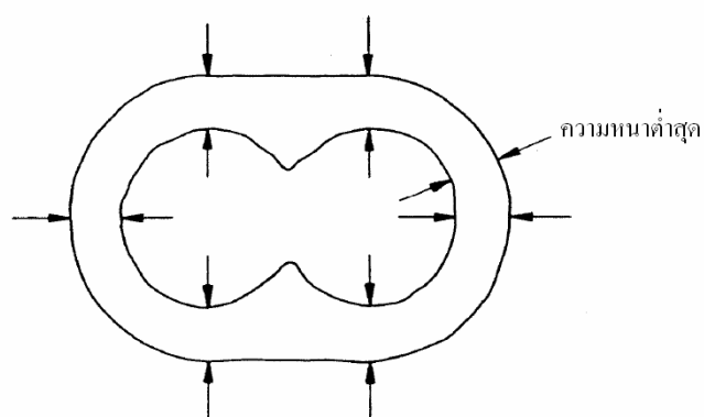
รูปที่ ก.10 (ก) แสดงการวัดค่าความหนาของเปลือก (สายแบบ 2 แกน)
