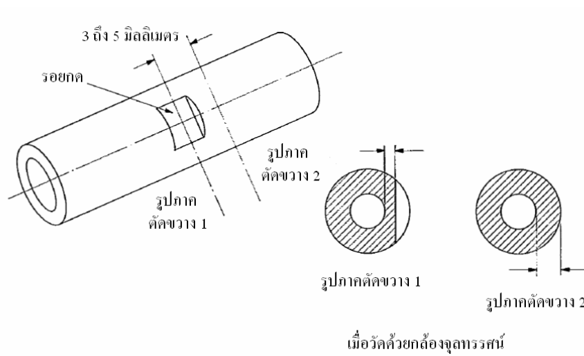
รูปที่ ค.3 การวัดรอยกดสำหรับขั้นตอนทดสอบที่มีขนาดเล็ก
