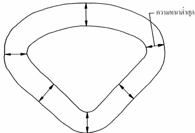
รูปที่ ก.2 แสดงการวัดค่าความหนาของฉนวน (ตัวนำรูปสามเหลี่ยมฐานโค้ง)
