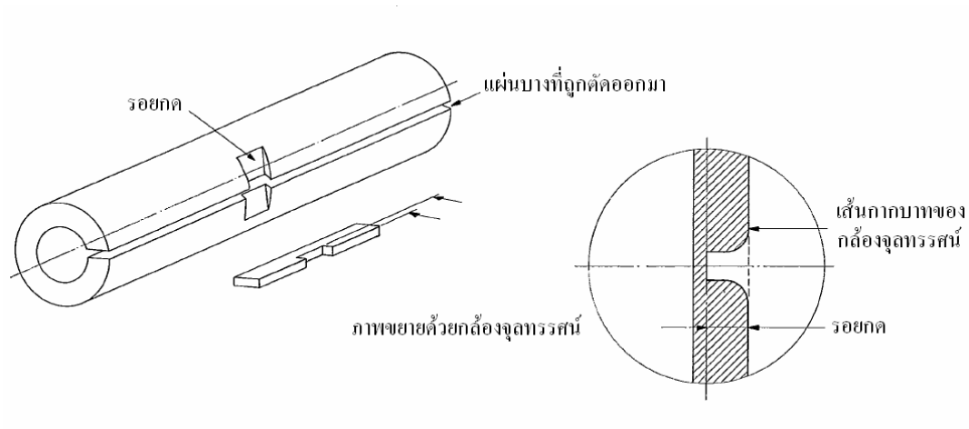
รูปที่ ค.2 การวัดรอยกด
