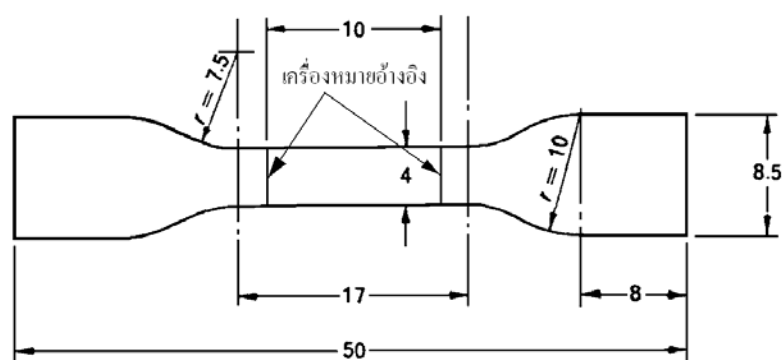
รูปที่ ก.13 แสดงขั้นตอนทดสอบรูปดัมเบลล์เล็ก
