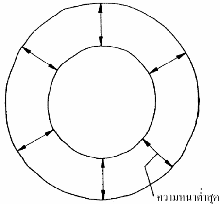
รูปที่ ก.1 แสดงการวัดค่าความหนาของฉนวนและเปลือก (หน้าตัดข้างด้านในที่เป็นวงกลม)
