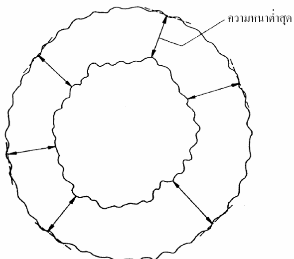
รูปที่ ก.5 แสดงการวัดค่าความหนาของฉนวน (หน้าตัดข้างด้านนอกไม่เรียบ)
