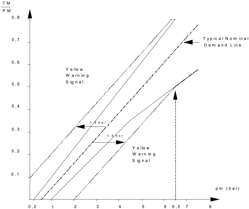
D I A G R A M 2 . T r a c t i v e U n i t s f o r S e m i - t r a i l e r s .
