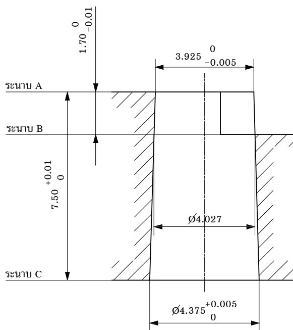
รูปที่ 4 มิติเครื่องมือวัดรูปกรวย ความเร็ว 0.06 : 1 (ข้อ 8.4.1.1)
