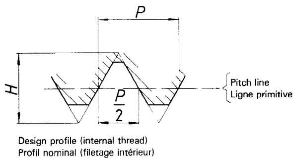
Figure 7 — Design profile for internal thread (Example) Figure 7 — Profil nominal pour filetages intérieurs (Exemple)
