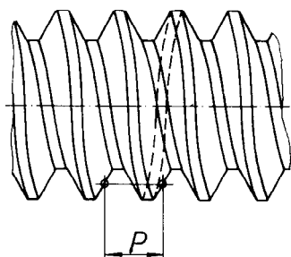
Figure 2 — Single-start right-hand external thread Figure 2 — Filetage extérieur à droite à un seul filet
