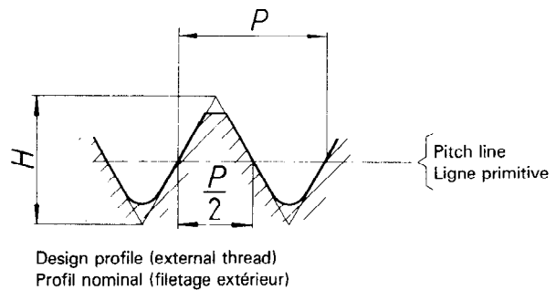
Figure 8 — Design profile for external thread (Example) Figure 8 — Profil nominal pour filetages extérieurs (Exemple)
