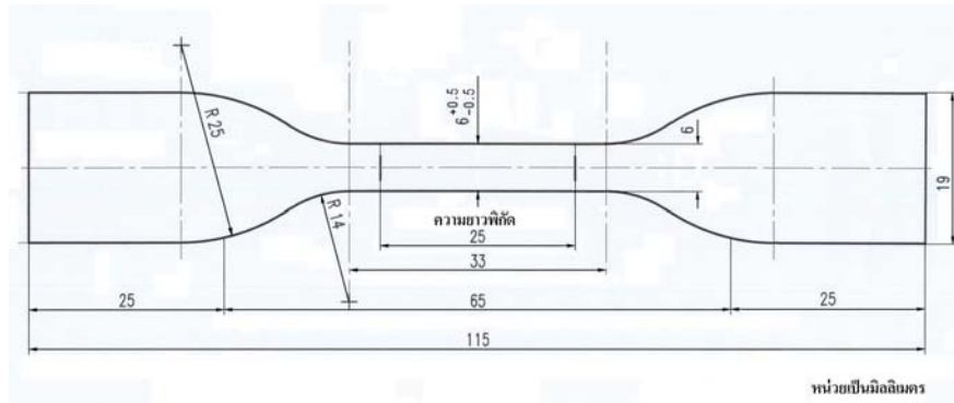
รูปที่ 2 ชั้นทดสอบรูปดัมพ์เบสล์ (ข้อ 10.8.2)
