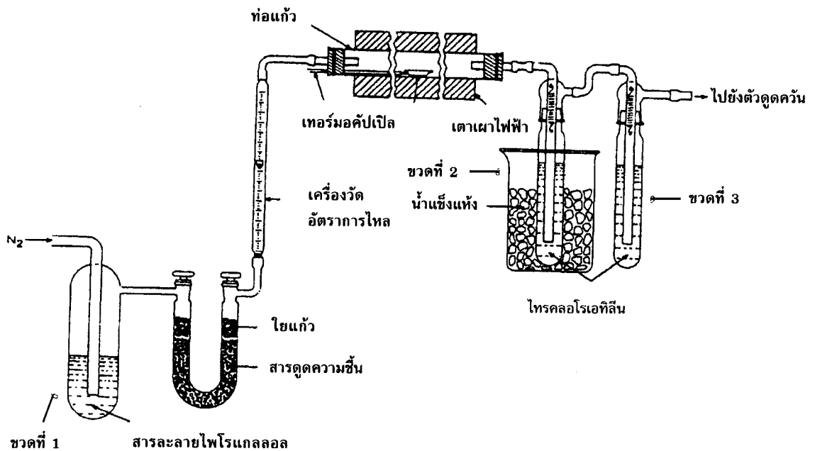
รูปที่ ข.1 การทดสอบปริมาณคาร์บอนแบล็กในเปลือกพอลิเอทิลีน
