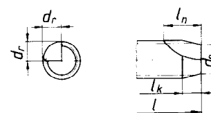
Scrape point Bout autonettoyeur Конец самонарезающего винта с притуплением
