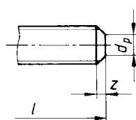
Flat point (chamfered point) Bout plat (chanfreiné) Плоский конец (с фаской)
