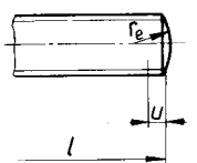
Rounded end Bout bombé Скругленный конец
