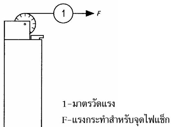
รูปที่ 3 การทดสอบการทำให้เกิดเปลวไฟสำหรับไฟแช็กแบบวงล้อตะไบขีดกับหินขีดไฟ (ข้อ 8.2.1)
